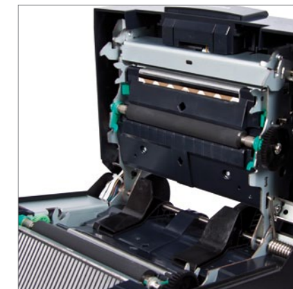
De DB-EA4D is uitgerust met een eenvoudig toegankelijke papierbaan, wordt onderhouden zonder gereedschap en heeft 2 thermische koppen om de voor- en achterzijde van direct thermische labels te bedrukken.
